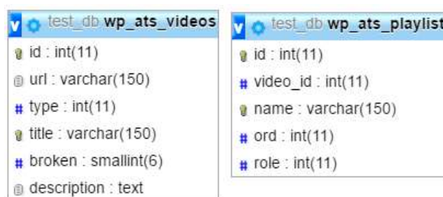
Obrázek 2: Přidané tabulky do databáze
