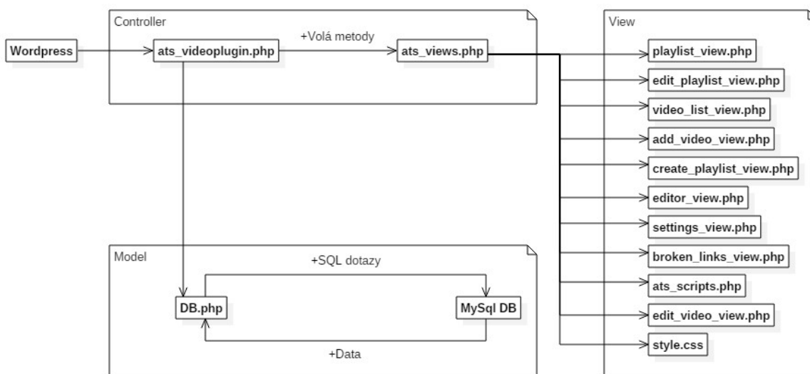
Obrázek 1: Schéma propojení komponent
